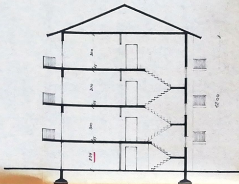
SEZIONE A-B
