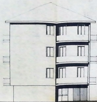
PROSPETTO NORD
