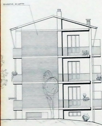
PROSPETTO EST
