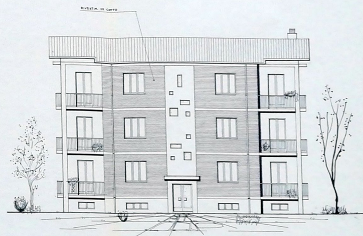
PROSPETTO SUD
